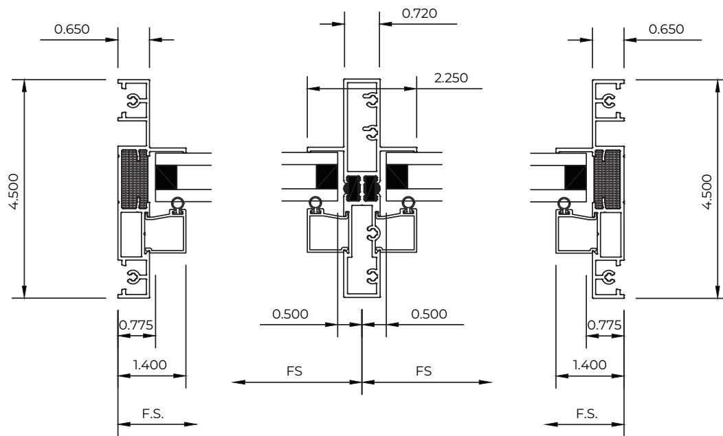
T-Bar Unit
